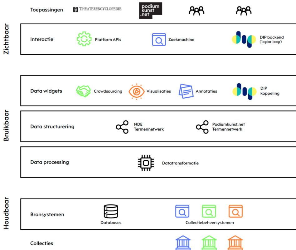
Figuur 1 Technische Architectuur
